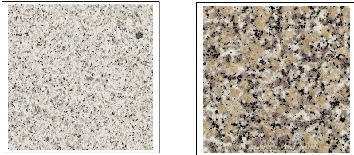
Figura 10. Variedades graníticas del plutón de La Cabrera en placas pulidas. A la izquierda, leucogranito de grano fino (variedad Blanco Berrocal ). A la derecha, monzogranito biotítico equigranular de grano medio (facies común) (variedad Crema Cabrera ). El aspecto rosado es debido a la alteración de minerales (óxidos de Fe-Ti) incluidos dentro de los cristales de feldespato potásico.
